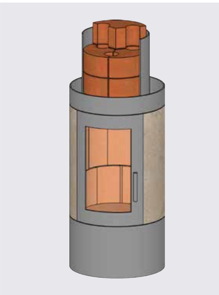
Камни аккумуляционного блока каминной печи
